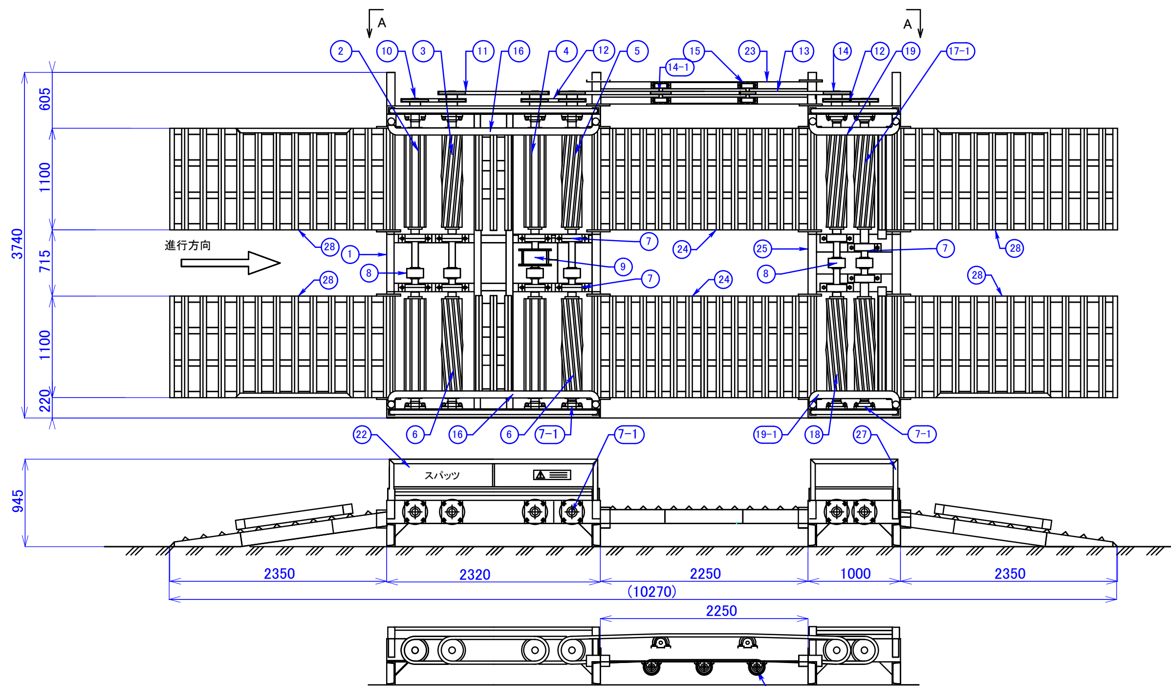
矢視 A-A
